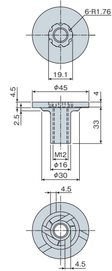
■寸法図
