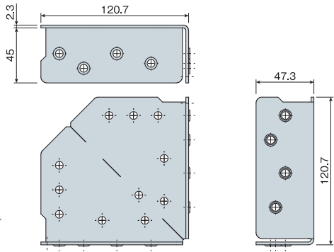
■寸法図
