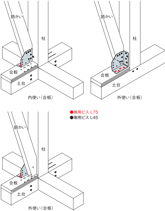
■取付図
