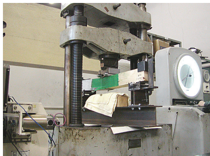
アラミド引張耐力試験(北海道大学 野口研究室)
