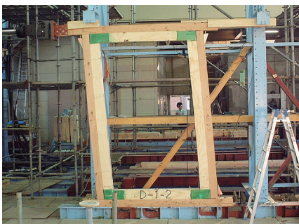
BOX型フレーム試験
